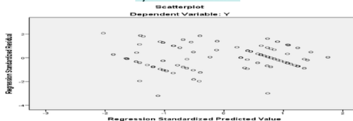
Gambar I Uji Heteroskedastisitas
