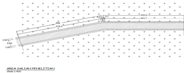
Gambar 4 Denah Pekerjaan Galian
