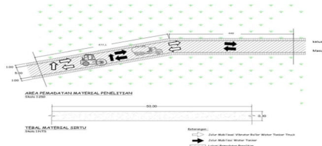
Gambar 3. Pelaksanaan Pematatan
