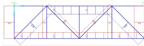
Gambar 6 Diagram Gaya – Gaya Dalam Model Rangka Jembatan Statis Tertentu
