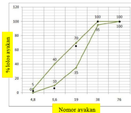
Gambar 4. Gradasi kerikil ukuran maksimum 40 mm
