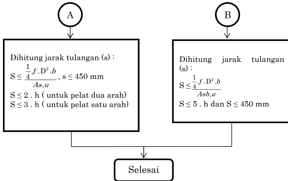
Gambar 1 Prosedur hitungan tulangan pelat (Sumber : Ali Asroni, 2010).
