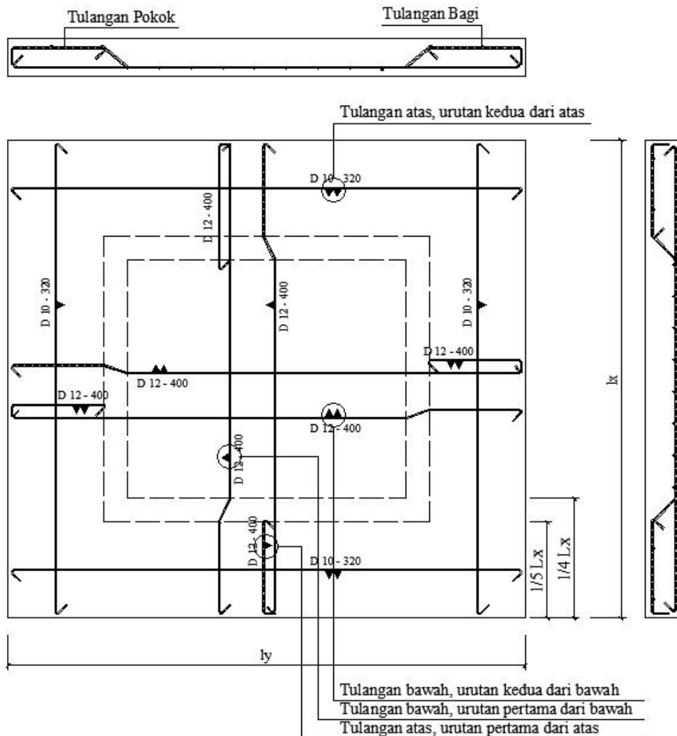
Gambar 5 Contoh pelat dengan penulangan dua arah
