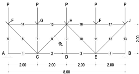
Gambar 5 Model Rangka Jembatan Statis Tertentu
