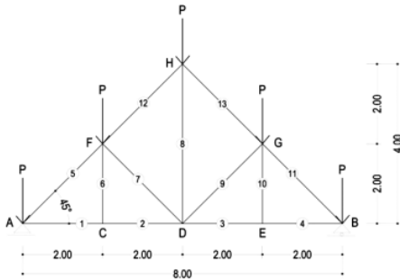
Gambar 1 Model Rangka Atap Statis Tertentu
