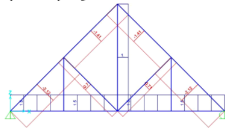
Gambar 4 Diagram Gaya – Gaya Dalam Model Rangka Atap Statis Tertentu
