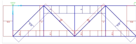
Gambar 6 Diagram Gaya – Gaya Dalam Model Rangka Jembatan Statis Tertentu
