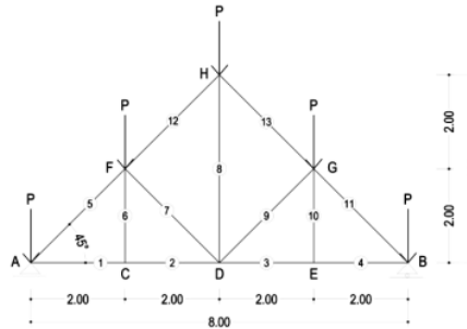
Gambar 3 Model Rangka Atap Statis Tertentu
