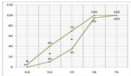
Gambar 3.9 Batas Gradasi Kerikil Ukuran 40mm.
