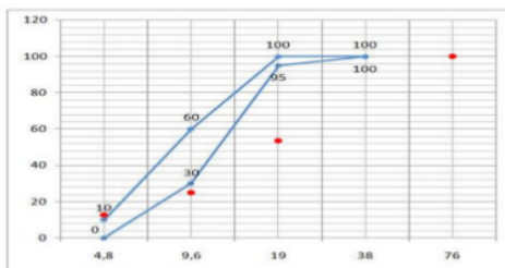
Gambar 3.8 Batas Gradasi Kerikil Ukuran Maksimum 20 mm
