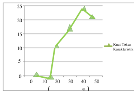
Gambar 3.10 Hubungan kuat tekan beton dengan penambahan limah serbuk besi dalam beberapa variasi.
