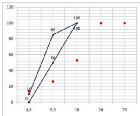
Gambar 3.7 Batas Gradasi Kerikil Ukuran Maksimum 10 mm
