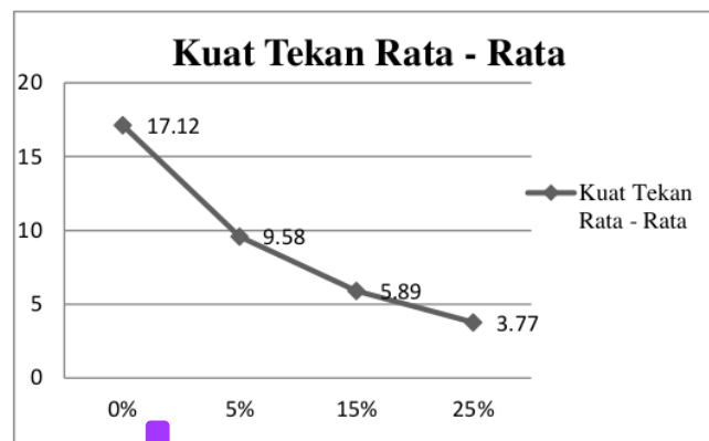
Gambar 2. Grafik Kuat Tekan Rata – rata
