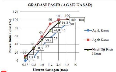
Gambar 2. Grafik Gradasi Pasir Hitam Masuk ke Zona 2
