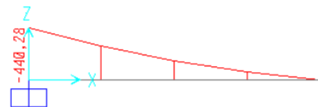
Gambar 8. Hasil Momen SAP 2000
