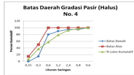
Gambar 7. Batas Gradasi Pasir Zona 4 Sumber: Hasil Pengolahan Data (2020)
