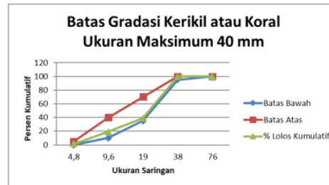
Gambar 10. Batas Gradasi Kerikil Ukuran Maksimum 40 mm Sumber: Hasil Pengolahan Data (2020)
