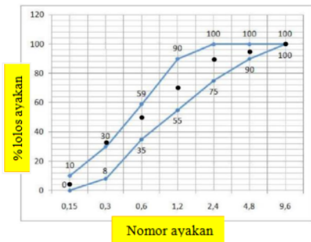
Gambar 3. Gradasi Pasir Zona 2
