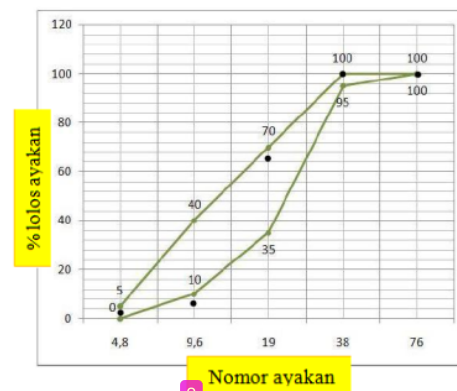
Gambar 4. Gradasi kerikil ukuran maksimum 40 mm
