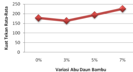
Gambar 5. Hubungan Kuat Tekan & Variasi Abu Daun Bambu
