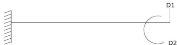
Gambar 2.12 Derajat Ketidak Tentuan Kinematis : 2
