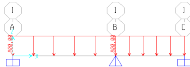
Gambar 2.47 Pemodelan Beban Merata
