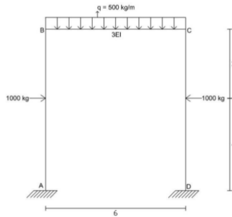
Lampiran 5. Struktur Portal yang dianalisa
