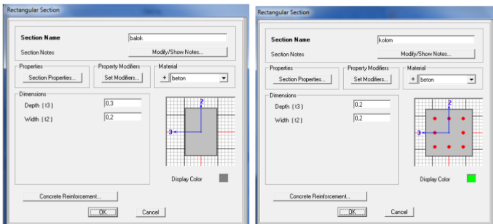
Gambar 2.49 Frame Section Balok & Kolom
