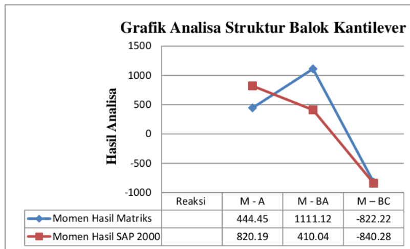
Lampiran 4. Grafik Analisa Struktur Balok Kantilever
