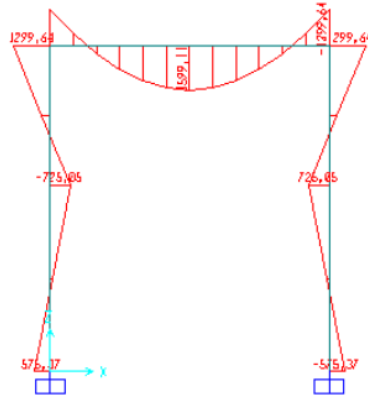
Gambar 2.52 Gaya Momen
