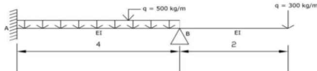
Gambar 2.17 Balok Kantilever Yang Akan Dianalisa
