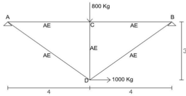
Lampiran 7. Struktur Rangka yang dianalisis
