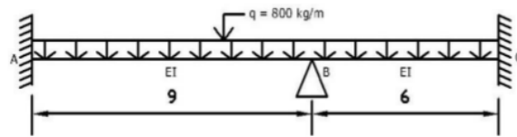
Lampiran 1. Struktur Balok yang dianalisa
