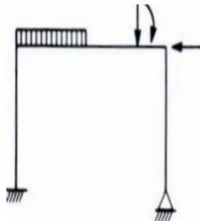
Gambar 1.4 Struktur Portal
