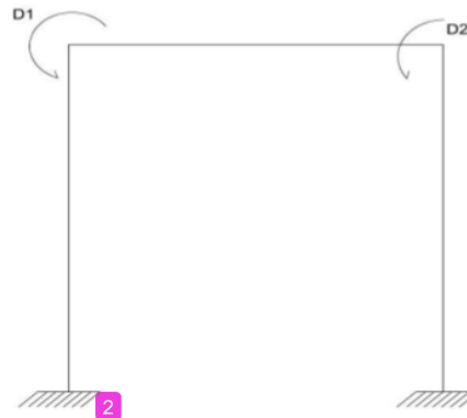
Gambar 2.29 Derajat Ketidak Tentuan Kinematis : 2
