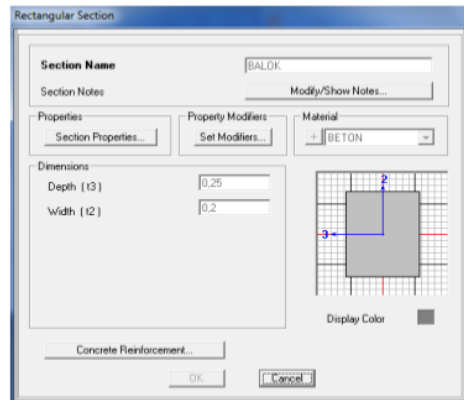
Gambar 2.57 Frame Section Balok Dan Kantiliver
