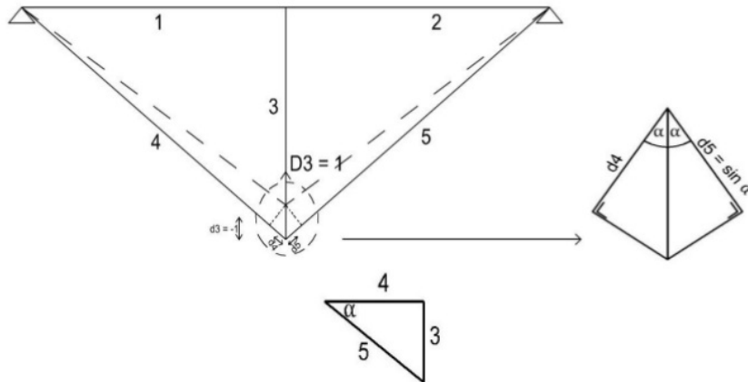
Gambar 2.41 Diberikan D_3 = 1 Satuan
