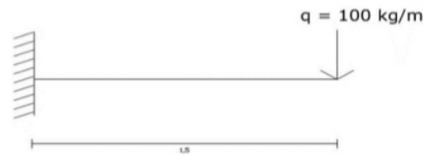
Gambar 2.10 Kantilever Yang Akan Dianalisa
