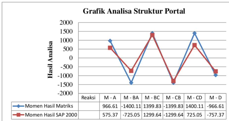
Lampiran 6. Grafik Analisa Struktur Portal
