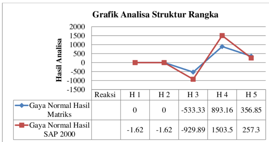
Lampiran 8. Grafik Analisa Struktur Rangka
