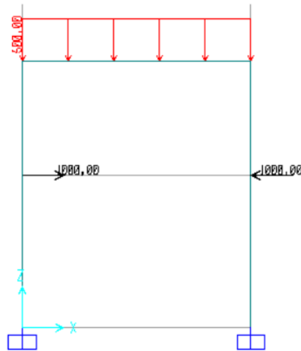
Gambar 2.51 Pemodelan Beban Pada Portal
