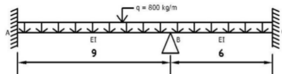
Gambar 2.1 Balok Yang Akan Dianalisa
