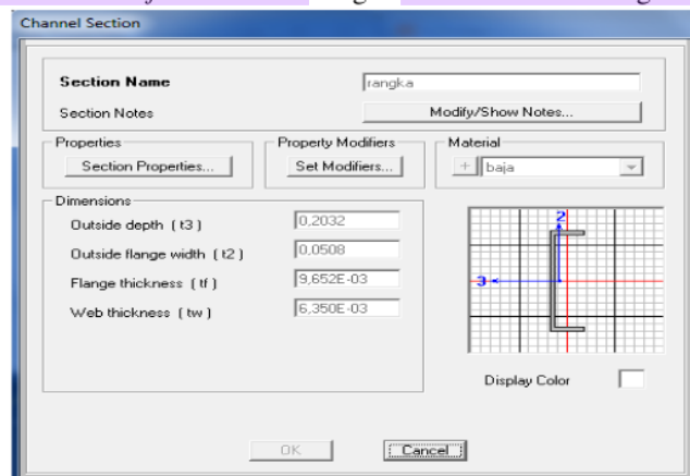
Gambar 2.53 Frame Section Rangka
