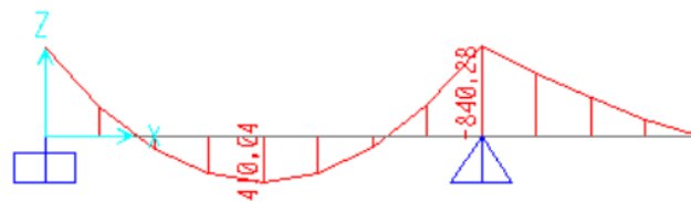
Gambar 2.60 Gaya Momen
