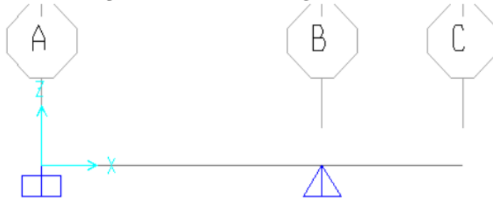
Gambar 2.58 Pemodelan Tumpuan Pada Balok Dan Kantilever
