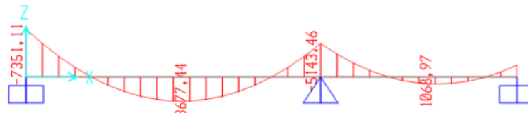
Gambar 6 2.48 Gaya Momen
