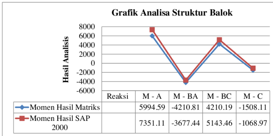
Lampiran 2. Grafik Analisa Struktur Balok
