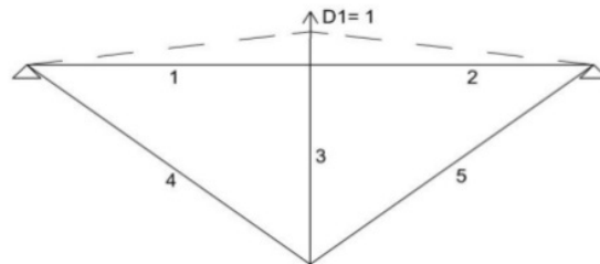
Gambar 2.39 Diberikan D1 = 1 Satuan
