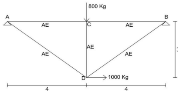
Gambar 2.35 Rangka Batang Yang Akan Dianalisa
