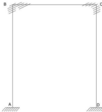
Gambar 2.27 Struktur Dasar Yang Dikekang
