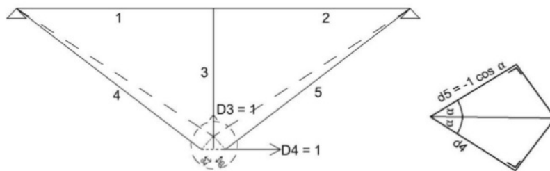
Gambar 2.41 Diberikan D_3 = 1 Satuan
