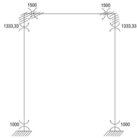
Gambar 2.28 Momen Primer
