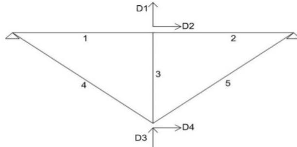
Gambar 2.37 Derajat Ketidaktentuan Kinematis : 4
