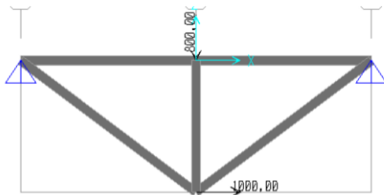
Gambar 2.55 Pemodelan Beban Pada Rangka
