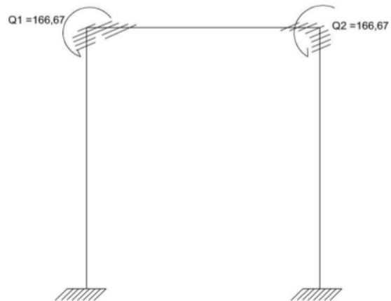
Gambar 2.30 Gaya Ekuivalen Dititik Diskrit Yang Koresponding Dengan Lentutan D
