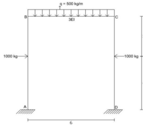
Gambar 2.26 Kontruksi Yang Akan Dianalisa
