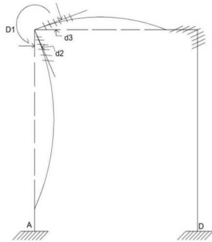
Gambar 2.31 Diberikan D_1 = 1 Satuan
