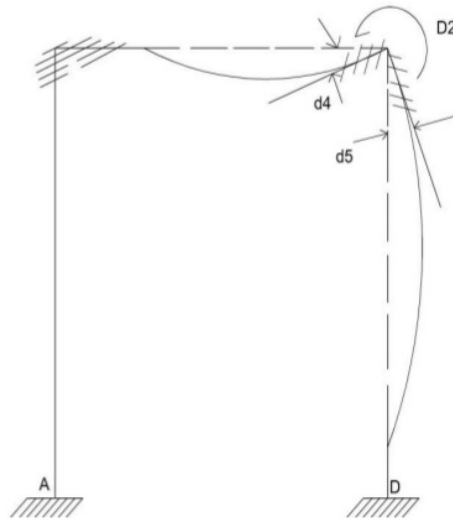
Gambar 2.32 Diberikan D_2 = 1 Satuan
