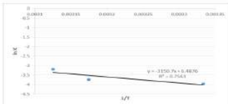
Gambar 4. Grafik hubungan antara nilai 1/T (K) dengan nilai \ln K pada produk kopi lengkuas instan.
