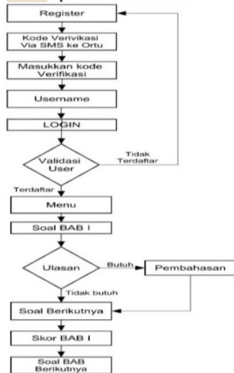
Gambar 2. Data Flow Diagram prototipe II untuk aplikasi “FunMath”
