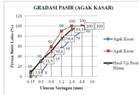
Gambar 2. Grafik Gradasi Pasir Hitam Masuk ke Zona 2
