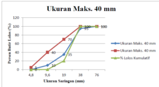
Gambar 3. Grafik Gradasi Agregat Kasar Ukuran Maksimal 40
