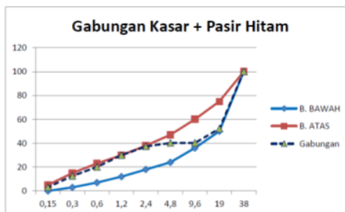
Gambar 4. Grafik Gradasi Gabungan Agregat
